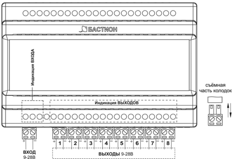
Рисунок 2 - общий вид изделия
