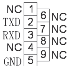
Назначение контактов разъема DB-9 (порт RS-232)
