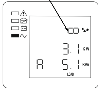
Рисунок 12 — ЖК-дисплей мощность нагрузки
