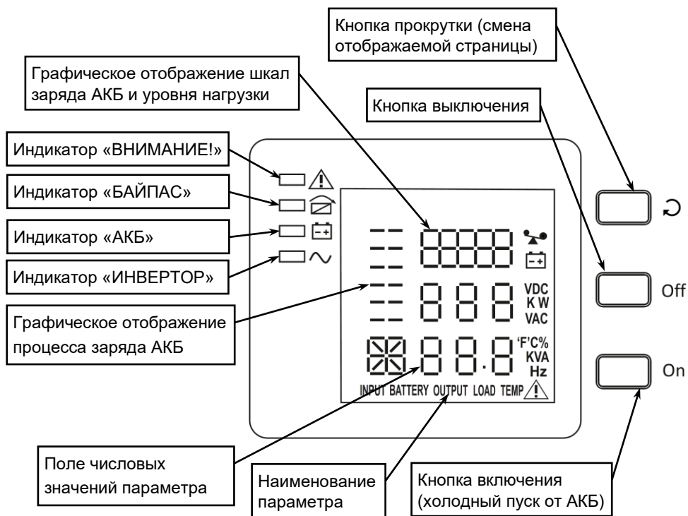
Рисунок 3 — Описание ЖК—дисплея
