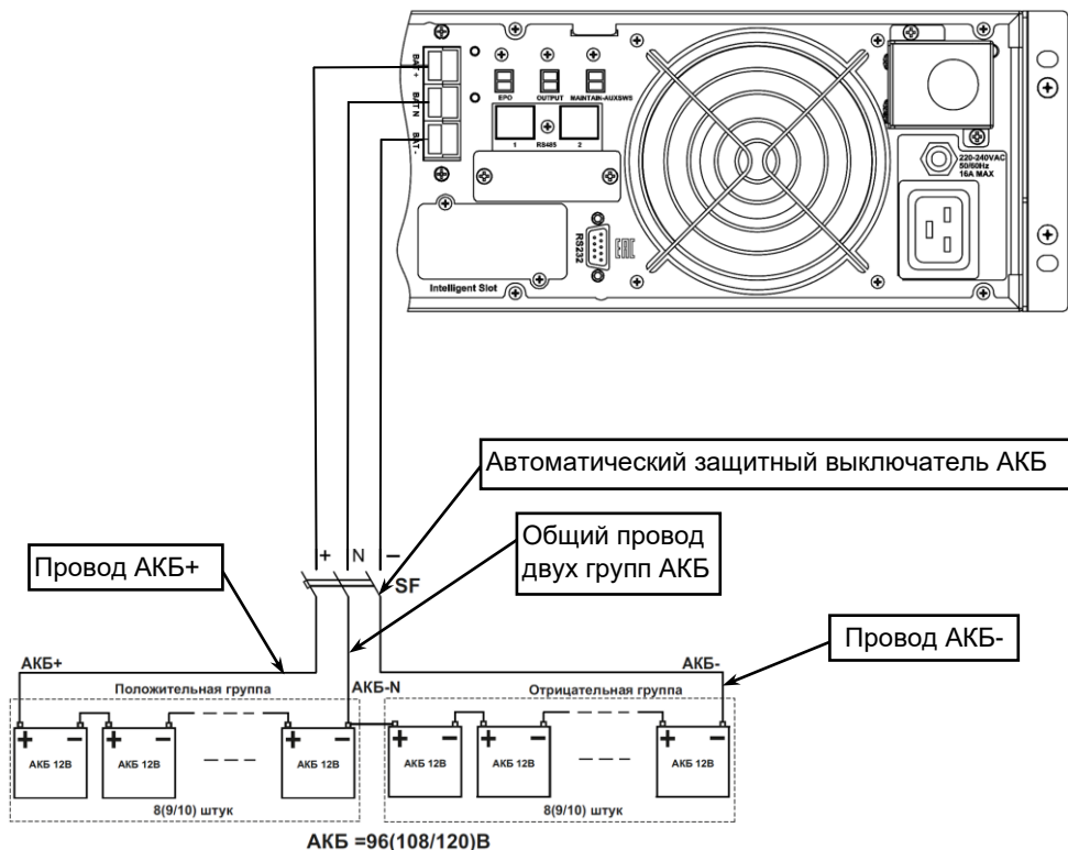
Рисунок 21 — Схема монтажа и подключения к ИБП аккумуляторной батареи.
